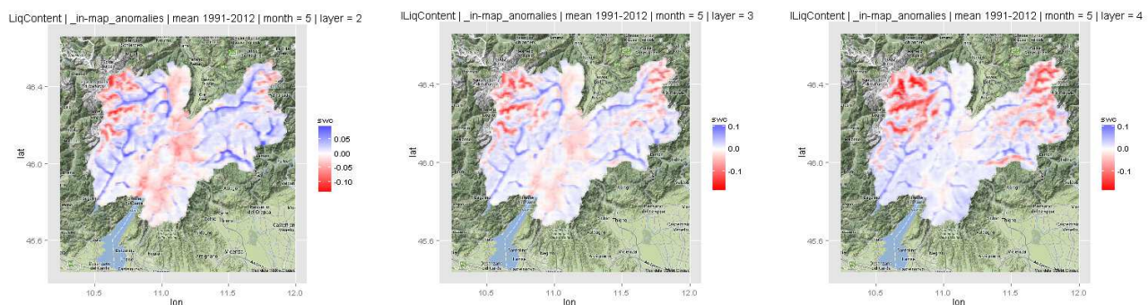
Fig. 13 - Contenuto medio di acqua nel suolo a tre profondità (da sinistra a destra: 8, 23 e 58 cm), mese di maggio, anomalie rispetto ai valori medi di mappa.
