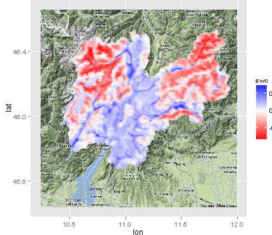
Fig. 10 - Come la Fig. 8, mappa delle differenze con i valori medi di mappa. Sinistra: aprile. Destra: luglio.
