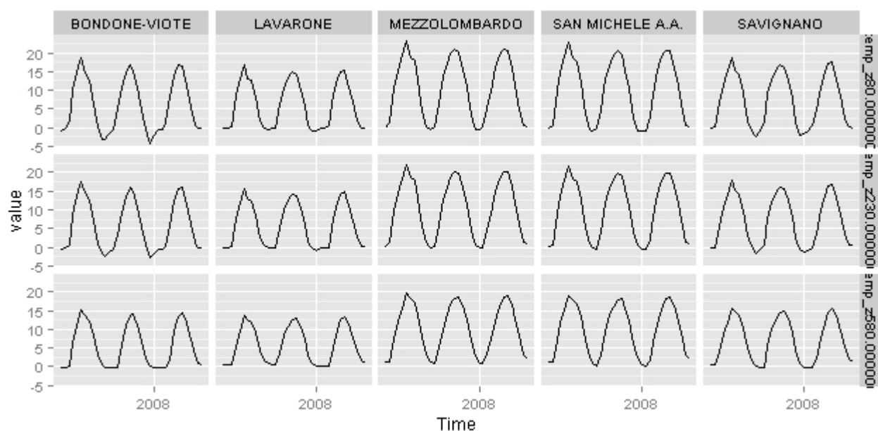
Fig. 4 - Simulazioni puntuali della temperatura media mensile del suolo [°C] per il periodo 2006-2008 in 5 posizioni di controllo. Prima riga: profondità media di 8 cm. Seconda riga: profondità media di 23 cm. Terza riga: profondità media di 58 cm.
