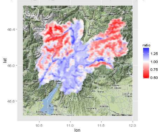
Fig. 11 - Come la Fig. 10, mappa dei rapporti con i valori medi di mappa
