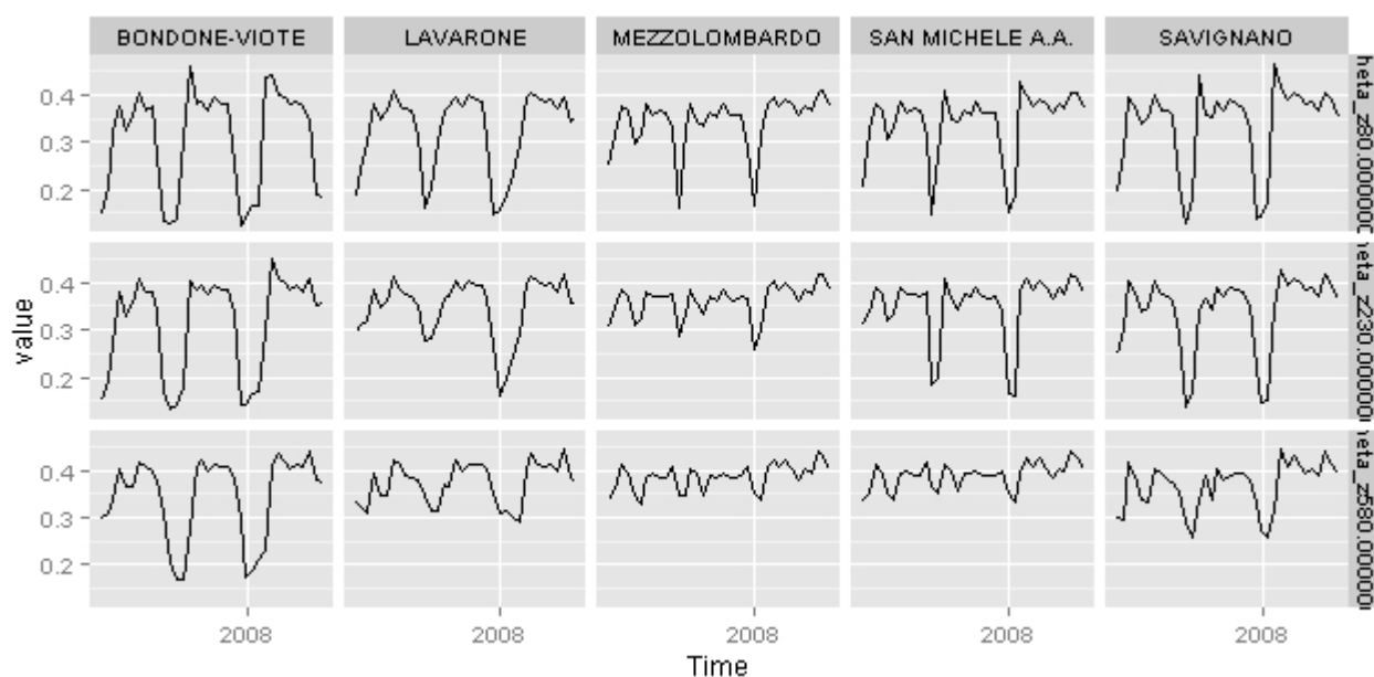
Fig. 6 - Simulazioni puntuali del contenuto d'acqua per il periodo 2006-2008 in 5 posizioni di controllo, a tre profondità crescenti: 8 cm, 23 cm, 58 cm (profondità media dello strato)
