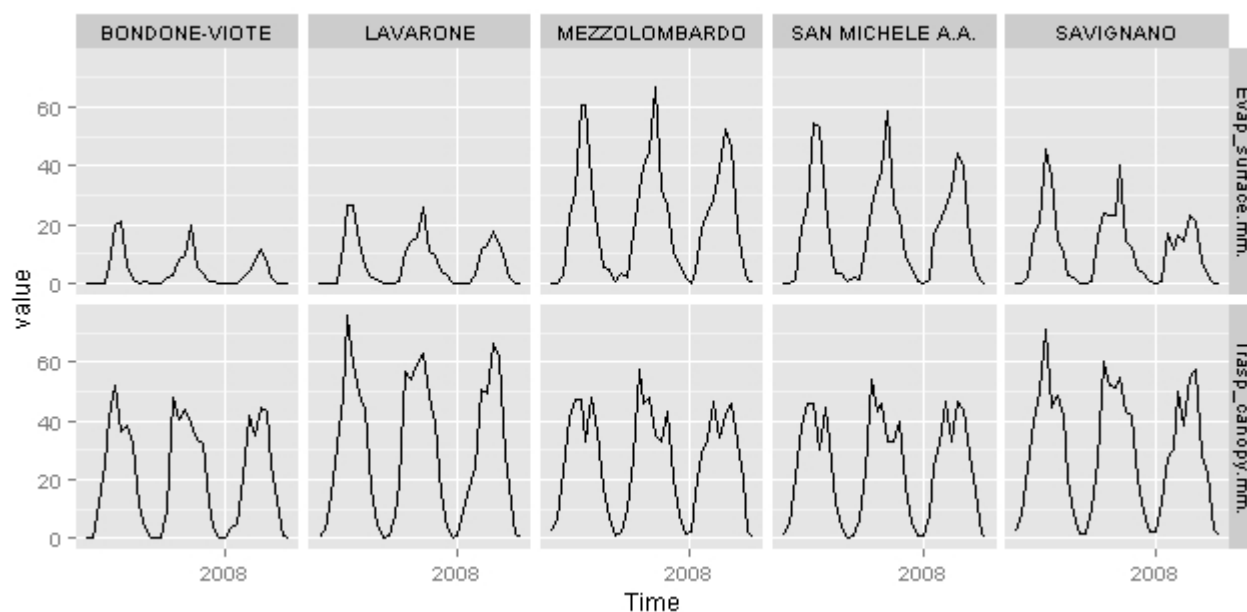
Fig. 5 - Simulazioni puntuali delle componenti di evapotraspirazione mensile [mm] per il periodo 2006-2008 in 5 posizioni di controllo. Prima riga: evaporazione dal suolo. Seconda riga: traspirazione dalla chioma.
