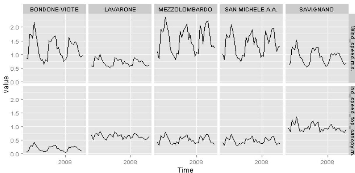
Fig. 3 - Simulazioni puntuali della velocità media del vento [m/s] per il periodo 2006-2008 in 5 posizioni di controllo. Pannelli superiori: velocità media. Pannelli inferiori: velocità alla sommità della chioma delle piante
