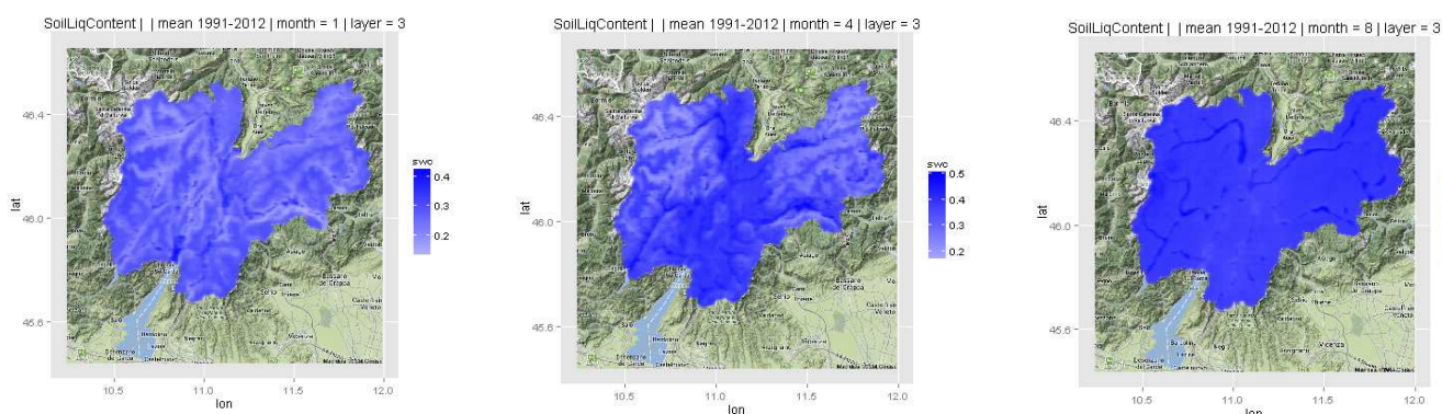
Fig. 8 - Contenuto medio di acqua nel suolo alla profondità media di 23 cm. Da sinistra a destra: gennaio, aprile, agosto.
