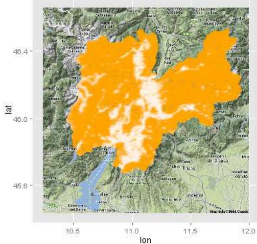
Fig. 15 - Carico di pressione sul suolo alla profondità media di 23 cm. Sinistra: aprile. Destra: luglio
