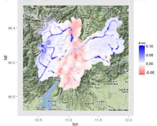
Fig. 10 - Come la Fig. 8, mappa delle differenze con i valori medi di mappa. Sinistra: aprile. Destra: luglio.
