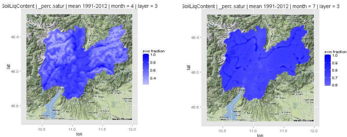
Fig. 9 - Contenuto medio di acqua nel suolo alla profondità media di 23 cm, valori riferiti al contenuto di acqua disponibile del suolo (frazione). Sinistra: aprile. Destra: luglio.
