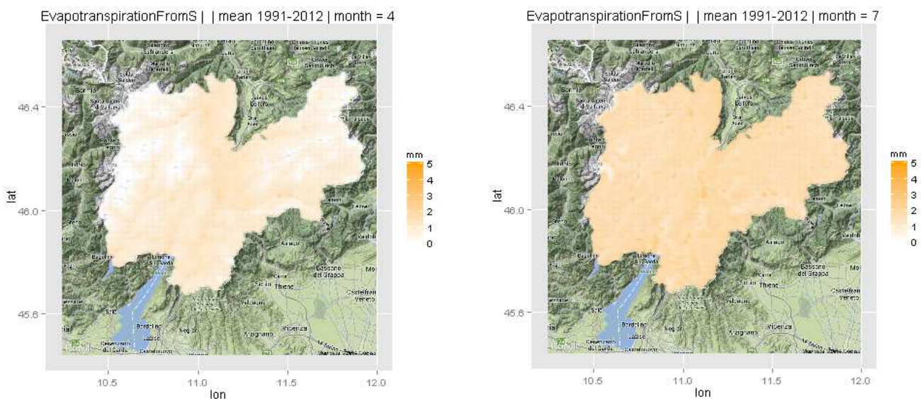
Fig. 16 - Mappe di evaporazione media dal suolo. Sinistra: aprile. Destra: luglio.
